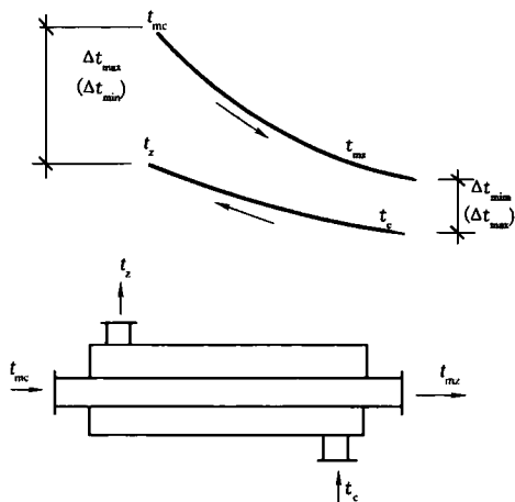
图6 快速水加热器水加热水工况示意
