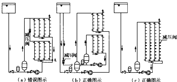
图 5 减压阀设置
