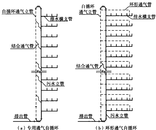
图 2 自循环通气模式
