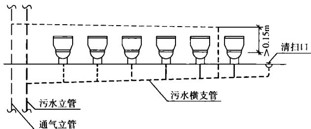
(b) 环形通气管与排水管及连接模式
