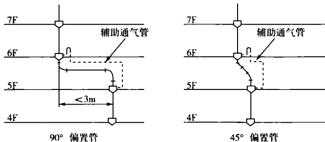
(d) 偏置管设置辅助通气管模式
