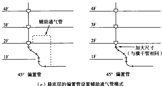
图 1 几种通气管与污水立管典型连接模式
